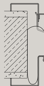
Steel case frame VarioFix
